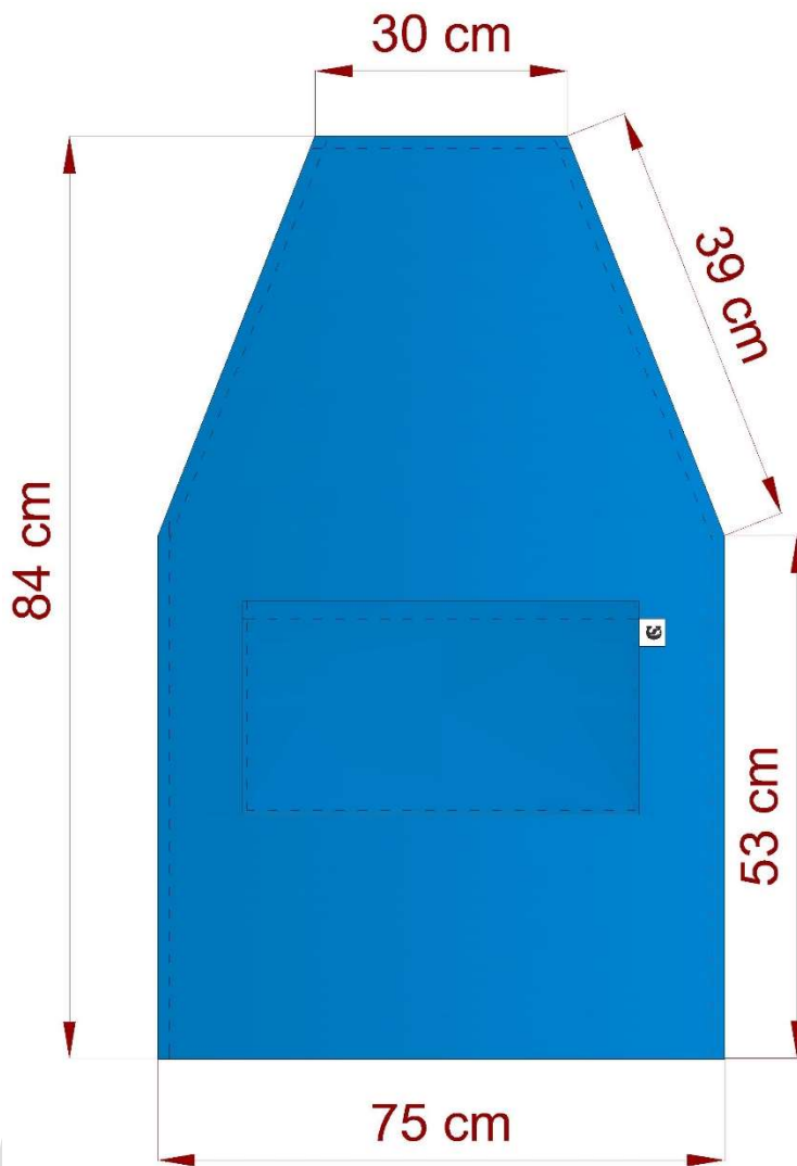
FIG. 1. MEDIDAS MANDIL PETO
